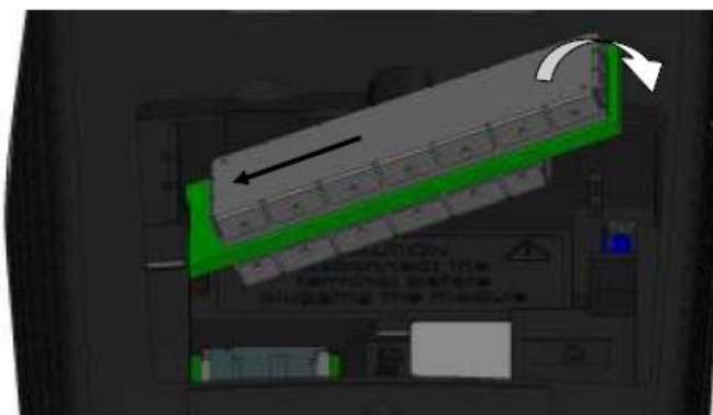
Рис. 6 Установка модуля считывания бесконтактных карт 2
