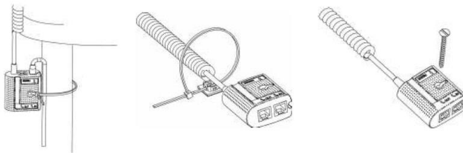
Рис. 10 Крепление кабеля
